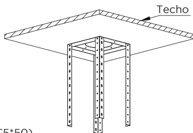
4 Tornillos (ST5*50) y 4 enchufes de pared
