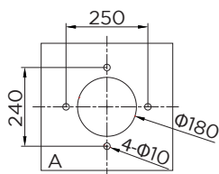
Tamaño de la posición del orificio de montaje
