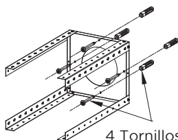
4 Tornillos (ST5*50) y 4 enchufes de pared
